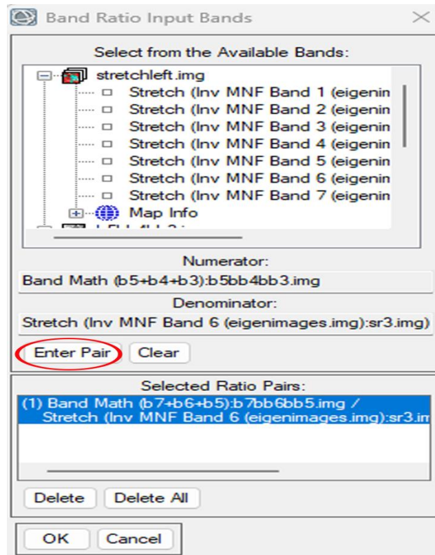
(Fig 3.2.5) using formula " ((b5+b4+b3)/b6) "
