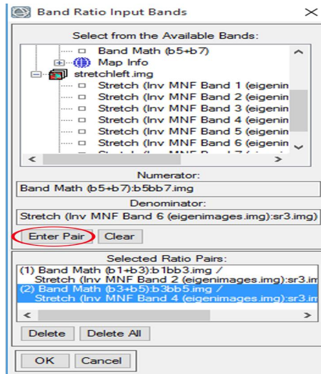
(Fig 3.3.6) using formula " ((b5+b7)/b6) "
